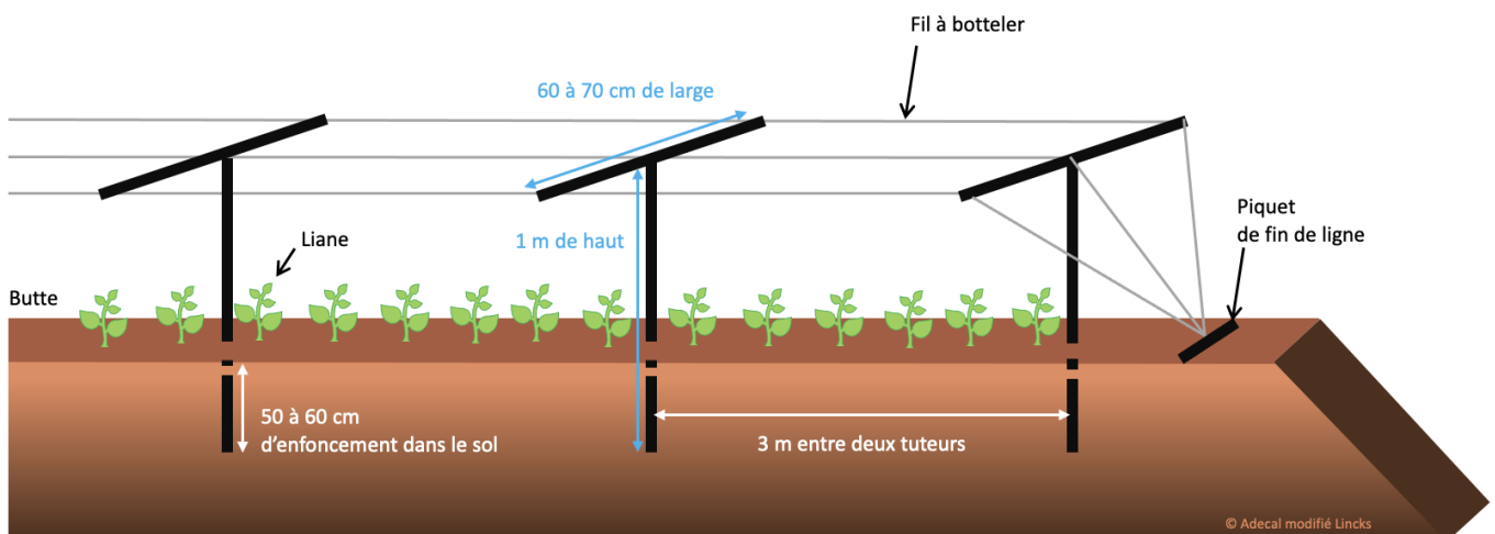
Schéma d'un tuteurage bas pour culture d'igname © Adecal modifié Lincks
